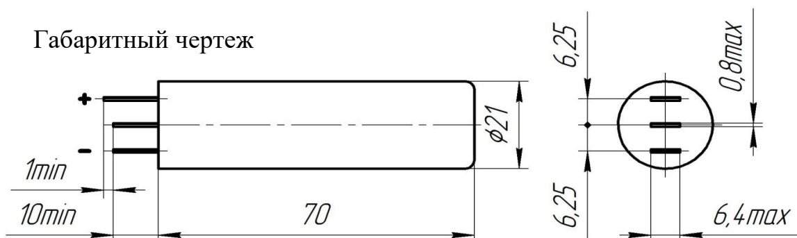
Нормально-замкнутый контакт
