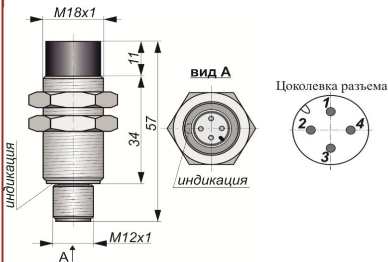
Габаритный чертеж
