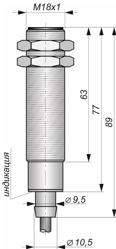
Габаритный чертеж
