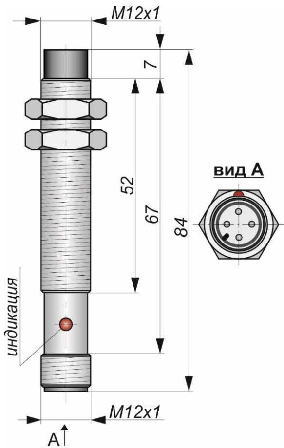
Габаритный чертеж
