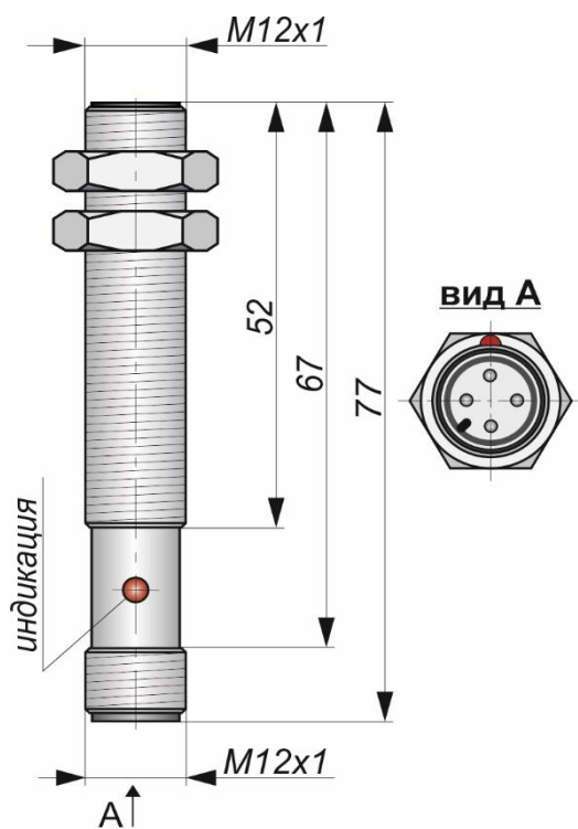
Габаритный чертеж
